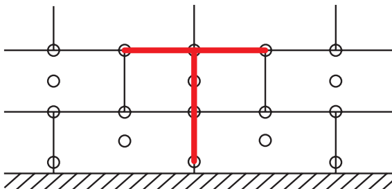
Т-дюбелиране при EPS-F
