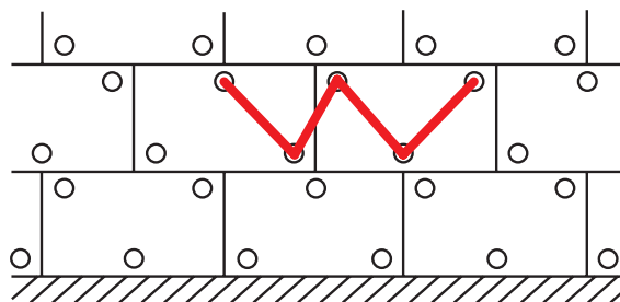
W-дюбелиране при минерална вата
