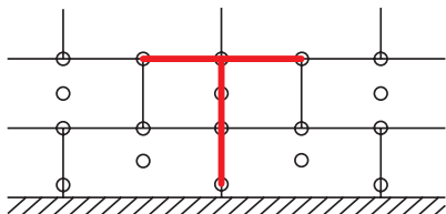
T-дюбелване при EPS-F
