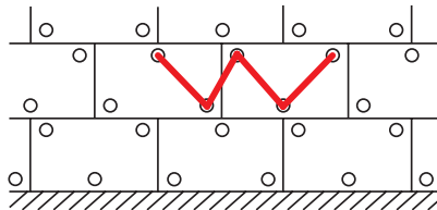
W-дюбелване при минерална вата
